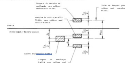
Figura 3 - Posições relativas das zonas de tolerância do diâmetro médio
