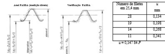
Figura 3 - Posições relativas das zonas de tolerância do diâmetro médio
